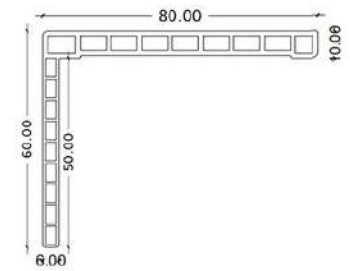
2 برواز 80 مم (8 سم) Scale 1:1
